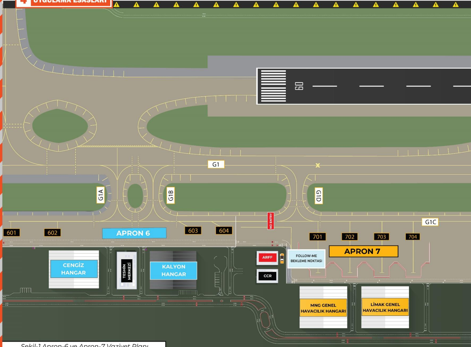
Şekil-1 Apron-6 ve Apron-7 Vaziyet Planı
