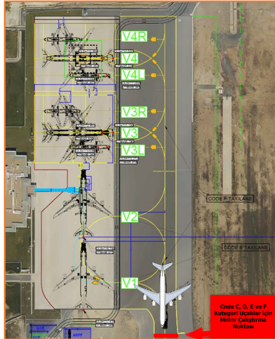
Şekil-2 Code C, D, E ve F Kategori Uçaklar için Gidiş - Departure Motor Çalıştırma Noktası
