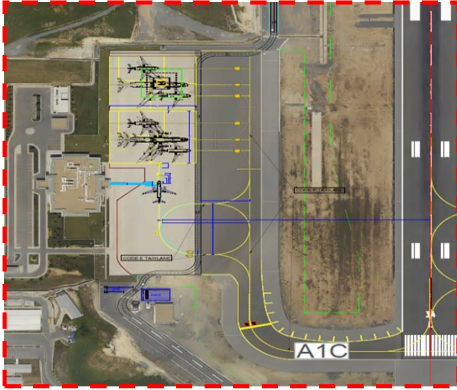
V Apronu - V1, V2, V3L, V3, V3R, V4L, V4, V4R Park Sahaları
